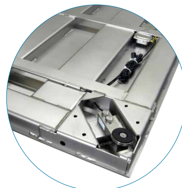
Detalle del alojamiento de la célula de carga
